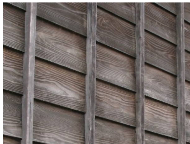
ささらこ状の押し縁による下見板の固定
